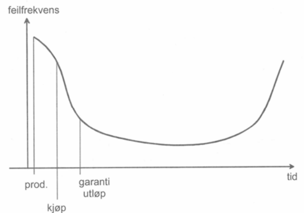
Figur 1: Sannsynlig feilfrekvens som funksjon av tid.
