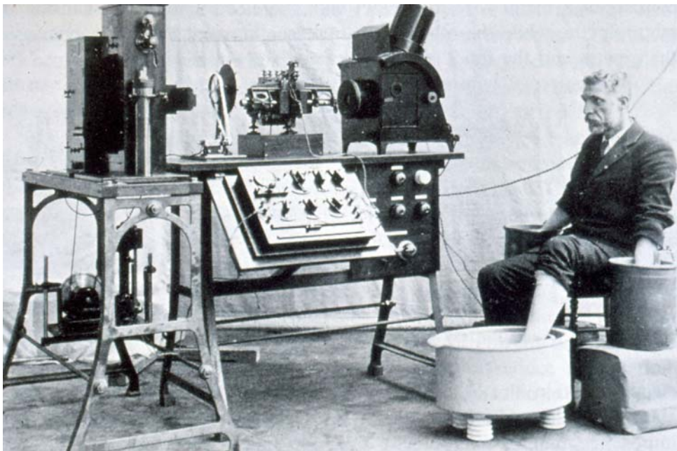
En registrering av hjertets elektriske aktivitet, elektrokardiografi – EKG, ble vist av Wilhelm Einthoven i 1905. Registreringssystemet var basert på et følsomt galvanometer som via optikk svertet en lysfølsom film. Registreringen er basert på de samme tre standard elektrodeforbindelser som ofte brukes i dag, begge armene og en fot. Kontakten med pasienten skjedde gjennom de tre saltvannsfylte bøttene – «elektrodenene». Registreringene ble nesten like bra som i dag, noe som skyldtes at lysnettet ennå ikke var utbredt og dermed ikke virket inn som elektrisk støykilde. Foto: Ukjent.
